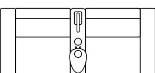
1B + SB CONSOLE (LAD. BRAÇO: DIREITO OU ESQUERDO) (BRAÇO: 15 OU 25CM) (FORM. CONSOLE: RETO OU ANGULAR) (COMP. CONSOLE: 25 OU 40CM) (LAD. CONSOLE: DIREITO OU ESQUERDO) 0,80 x 1,12 m | 31 4/8 in x 44 1/8 in 0,90 x 1,12 m | 35 3/8 in x 44 1/8 in 1,10 x 1,12 m | 43 2/8 in x 44 1/8 in
